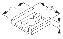
SG 10865 Montageplatte
