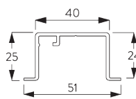
SG 10862 Nutprofil
