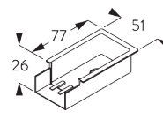
SG 10864 Nutmaske
