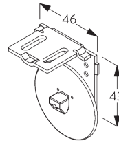
SG 11198 Träger
