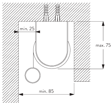
Träger SG 10873
